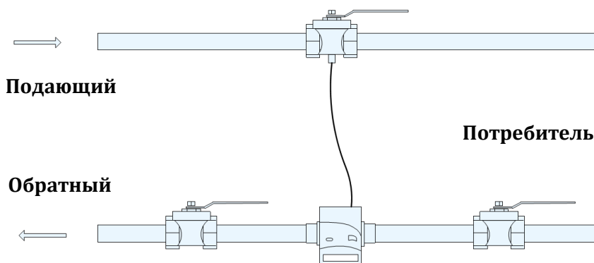
Рисунок 9 - Установка теплосчетчика и температурных датчиков для Zelsius® C5-IUF на обратный трубопровод
