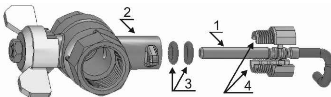
Рисунок 12 - Вариант установки термопреобразователя в шаровый кран
