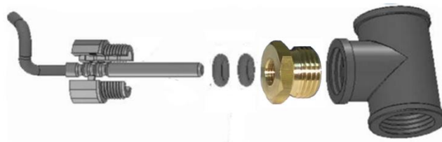
Рисунок 11 - Вариант установки термопреобразователя в тройник при помощи переходника.
