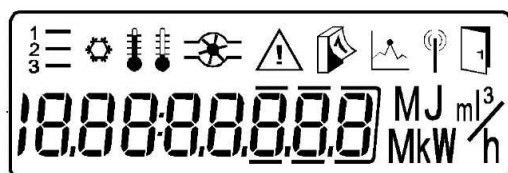
Рисунок 1 - Информационные поля ЖК-дисплея теплосчетчика
